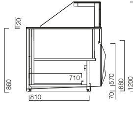
BDSNT balcão neutro com vidros counter neutral with glass comptoir neutre avec vitre contador neutro con vidrio
