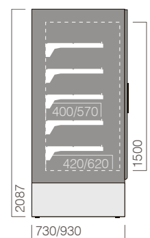
MF2 700 / 900N CP 3L1 murais multi deck -18°... -15° C
