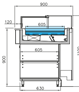
VMIND - VDB UV ventilada bitemperatura dual-temperature ventilated ventilée dual-temperature ventilada dual-temperatura
