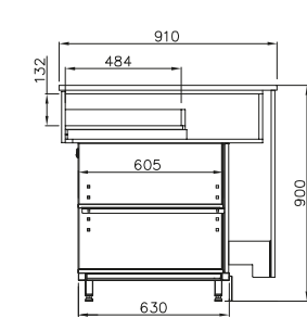
CX1N MIN B caixa support counter caisse caja
