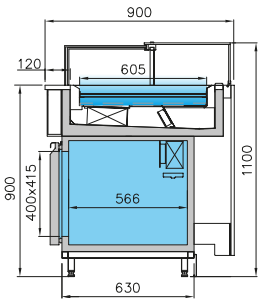
VMINVT - VDB UV 3M2 ventilada total total ventilated ventilée total ventilada total
