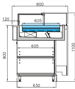
VMINVT - VDB UV 3M2 ventilada superior upper ventilated ventilée supérieure ventilada superior
