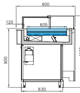
VMINVSCHR - VDB UV 3M2 vent. c/ sistema de humificação vent. w/ humidification system vent. avec système du humidification vent. c/ sistema de humificação
