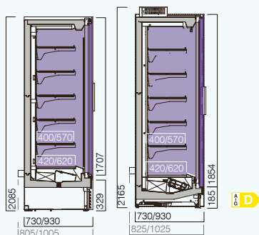
MF2 700/900 N CP FV - CG 3L1 (-18...-15 °C)
