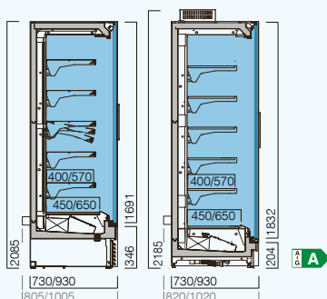
MF2 700/900 P CP FV - CG 3M1 (-1...+5 °C) 3M2 (-1...+7 °C)
